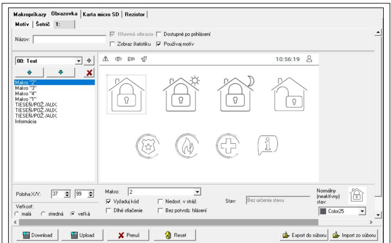
Obr. 17. Program DLOADX: záložka zobrazujúca obrazovku užívateľa (továrnske nastavenia).
