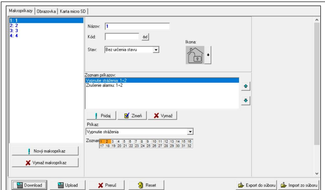
Obr. 24. Program DLOADX: klávesnica v systéme VERSA – záložka „Makropríkazy“ (príklad nastavení).
