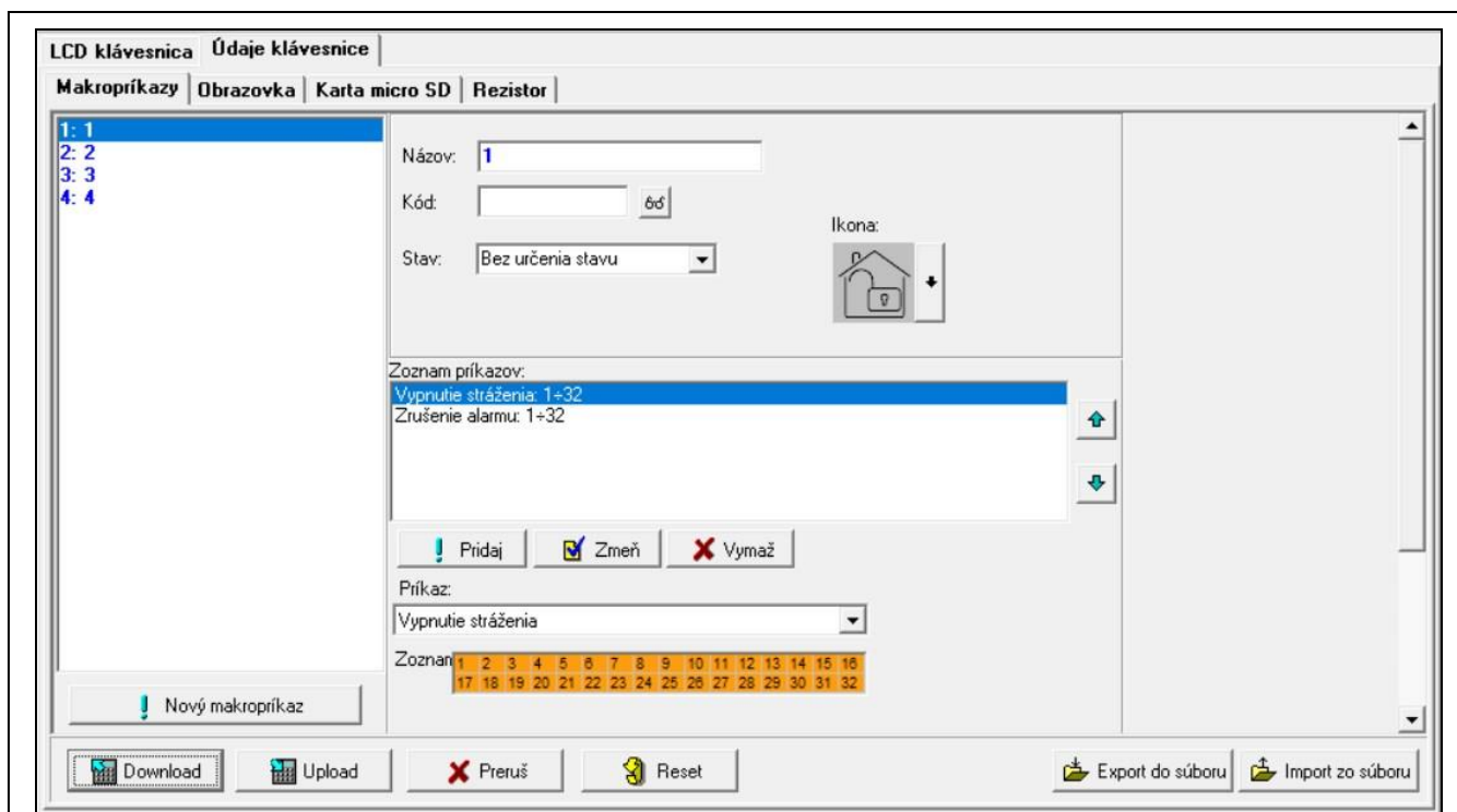
Obr. 14. Program DLOADX: klávesnica v systéme INTEGRA – záložka „Makropříkazy“ (továrenské nastavenia).
